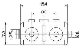
P板开孔图
