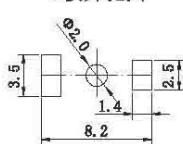
P板开孔图
