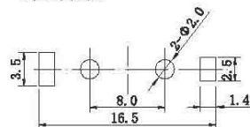
P板开孔图
